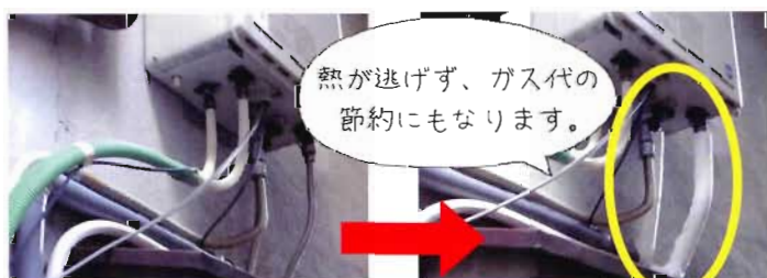
保温筒取り付け ～前～
