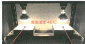
一般塗料塗布 表面温度48℃ ガイナ塗布 表面温度33.6℃
