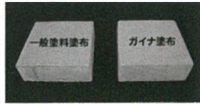
←一般塗料塗布コンクリートとガイナ塗布コンクリートを用意、コンクリートの厚みは50mm。それぞれを実験機に設置し、一般塗料塗布コンクリートの表面温度が48℃になるようライトを照射して、それぞれの裏面温度を計測。
