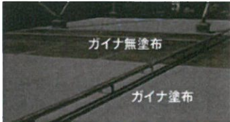
←RC造建築物上のガイナ塗布箇所とガイナ無塗布箇所表面温度を計測(測定日2006年9月3日、外気温:33℃)
