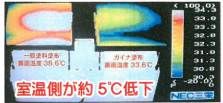
↑一般塗料塗布コンクリートの裏面温度は38.6℃、ガイナ塗布コンクリートの裏面温度は33.6℃となった。
